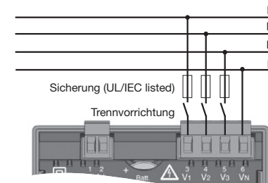
Anschlussvariante 3p 4w Spannungsmessung (Adr. 509 = 0, Standardeinstellung)
