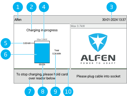
Abbildung 3.3: Anzeige während des Ladens an einer Steckdose
