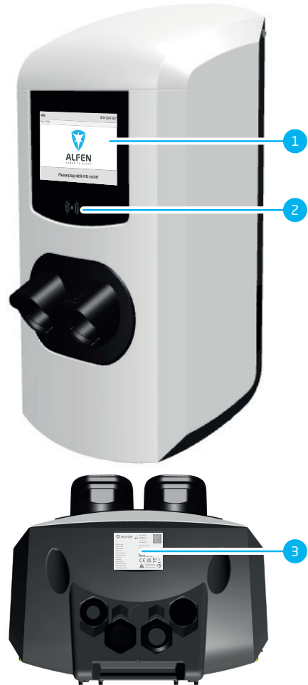
Abbildung 3.2: Modell mit fest installierten Ladekabeln (Kabel nicht abgebildet)
