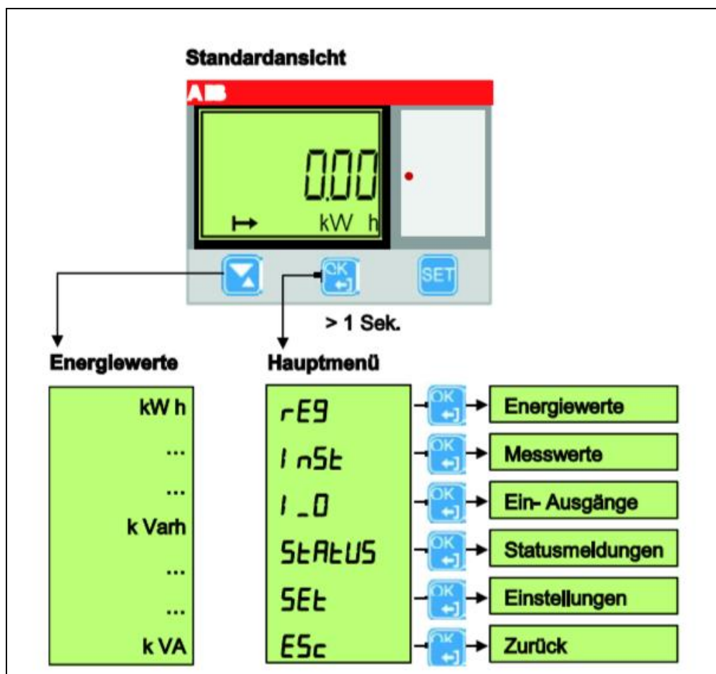
Abb. 7: Menüführung
