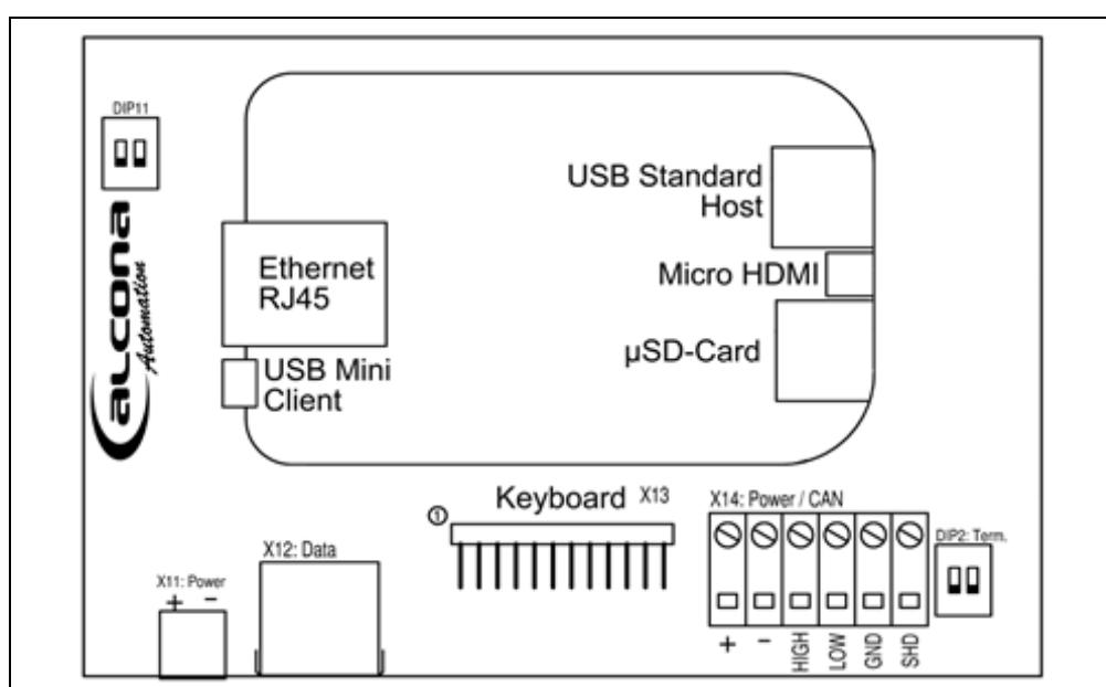
Abb. 2: Prozessorboard
