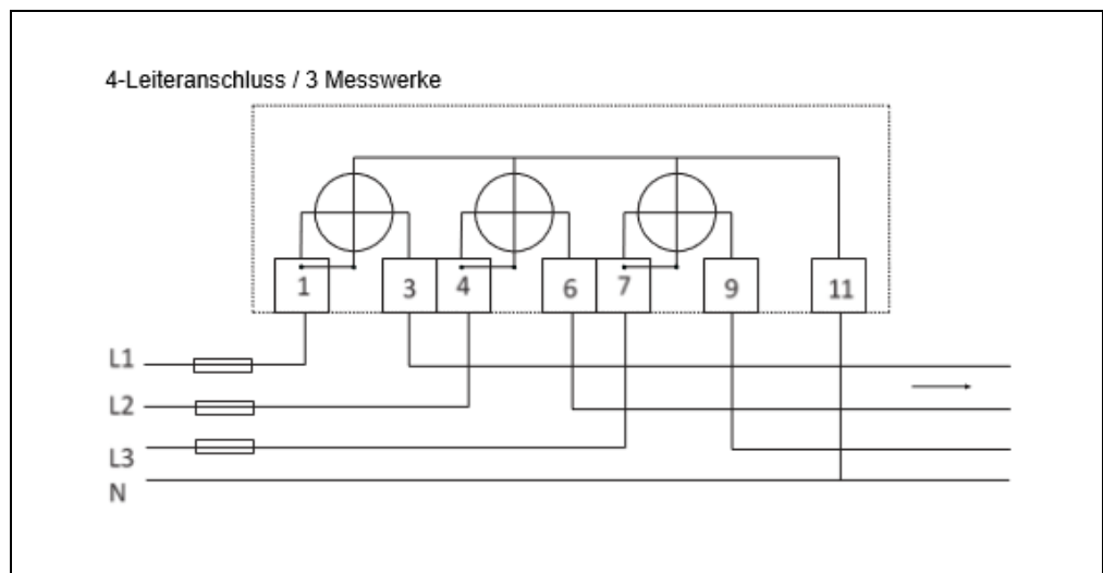
Abb. 5: Schaltbild
