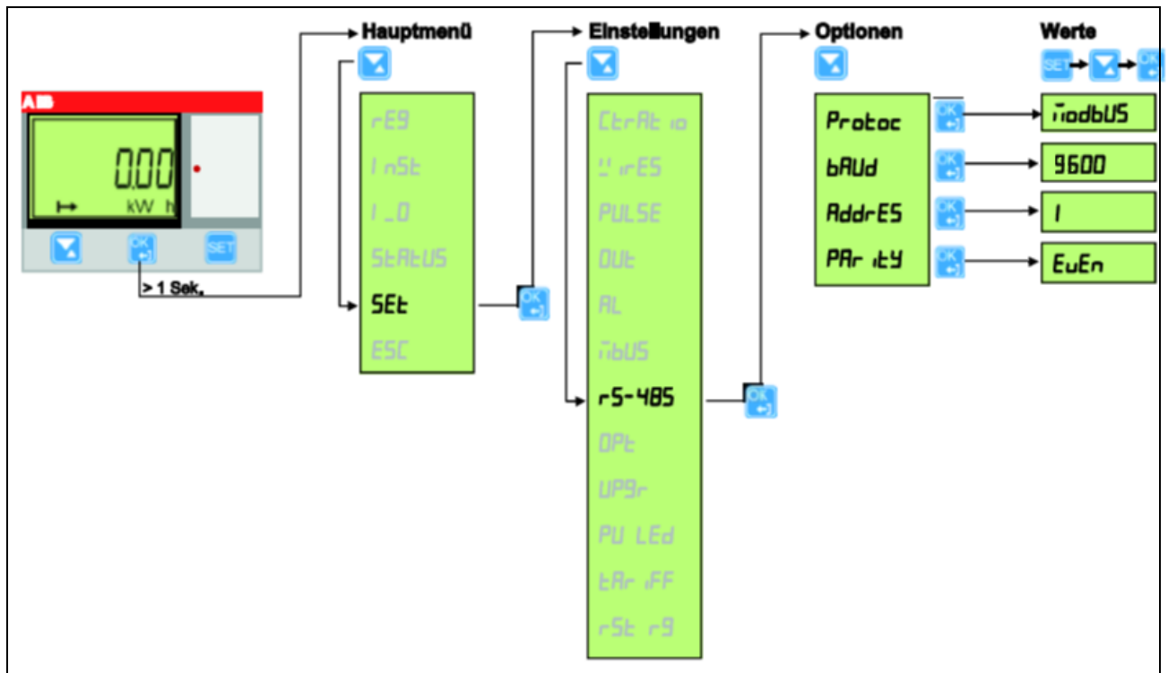
Abb. 8: Parametereinstellungen
