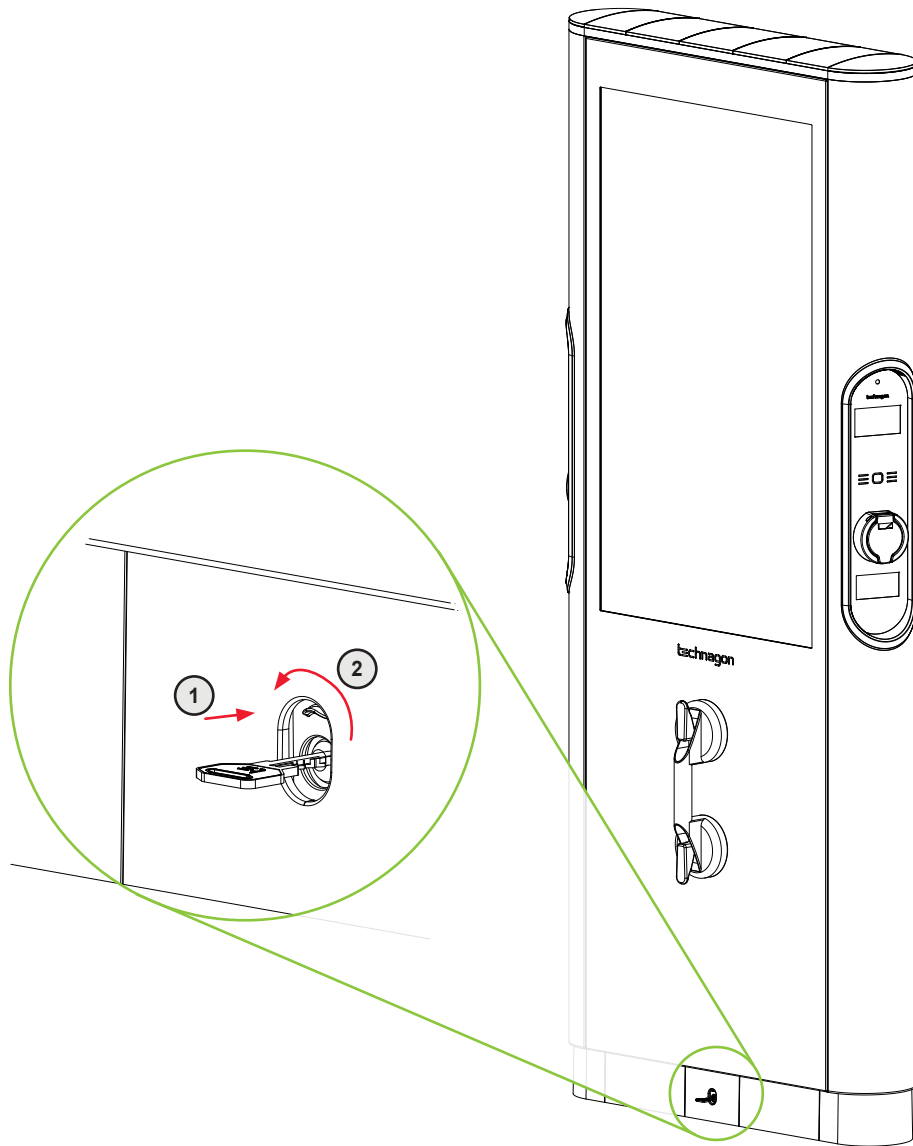
Abbildung 10: Gehäuse öffnen Technagon P80 – Frontblende/Türe entriegeln
