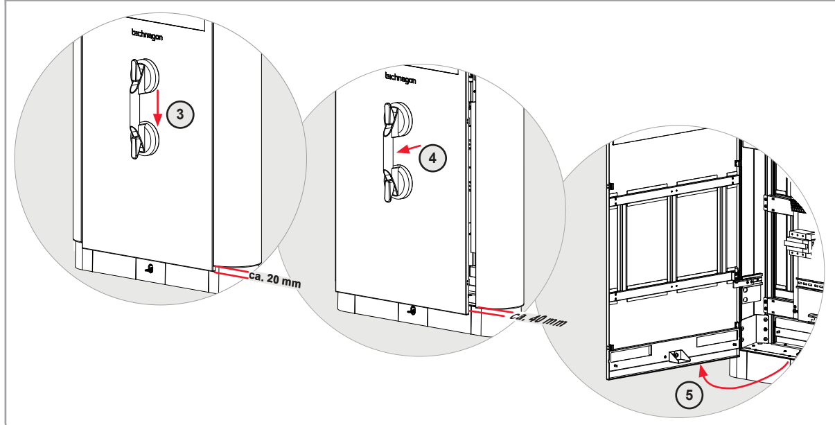
Abbildung 12: Gehäuse öffnen Technagon P80 – Anlagen mit schwenkbarer Türe
