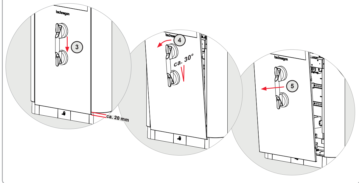
Abbildung 11: Gehäuse öffnen Technagon P80 – Anlagen mit abnehmbarer Frontblende
