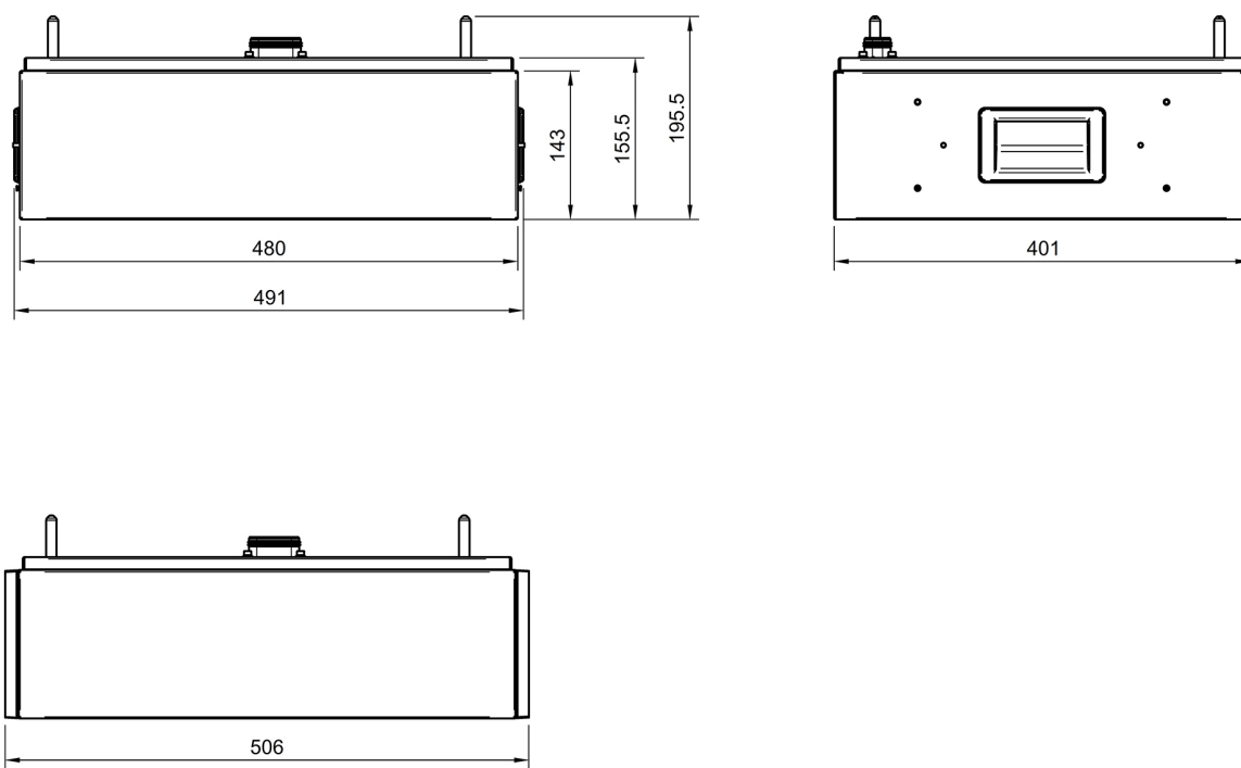
Abbildung 9. Abmessungen — Batteriemodul
