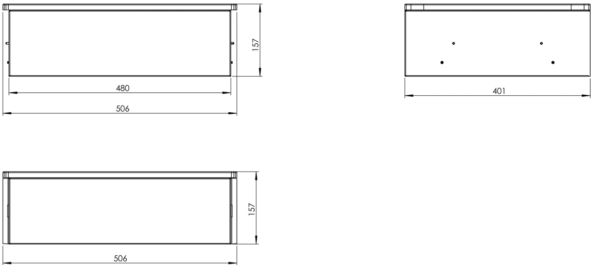
Abbildung 6. Abmessungen — Extension-Box
