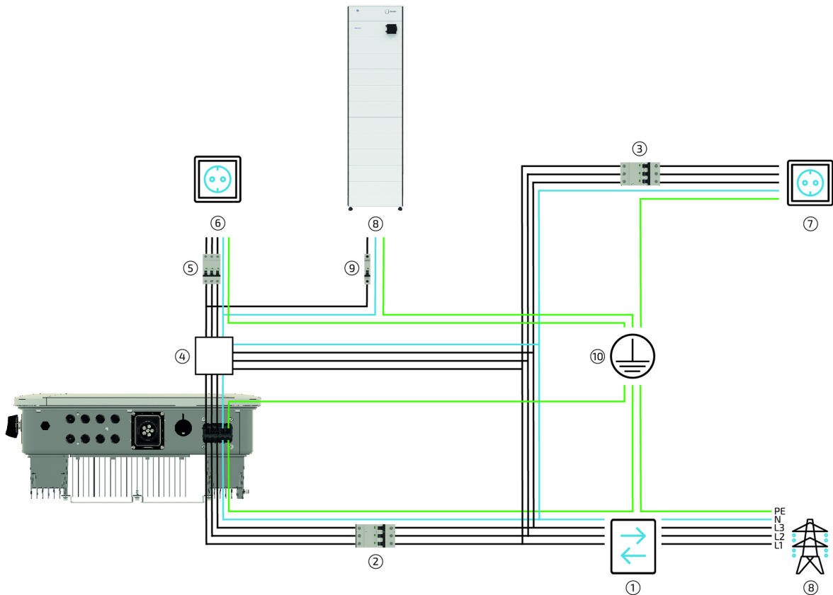
Abbildung 24. AC-Anschluss allgemein
