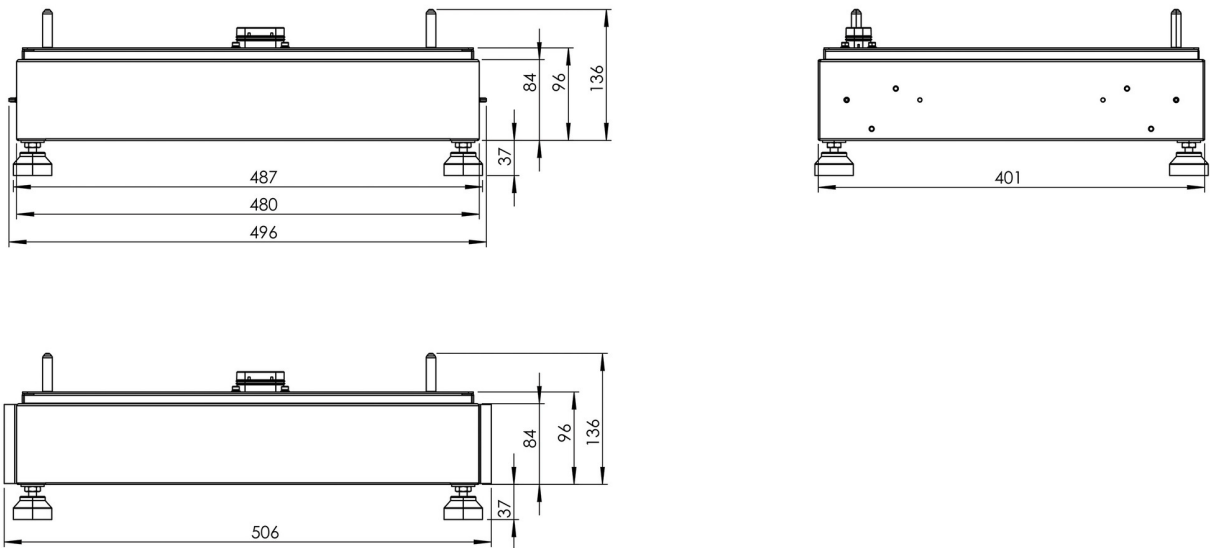
Abbildung 10. Abmessungen — Sockel
